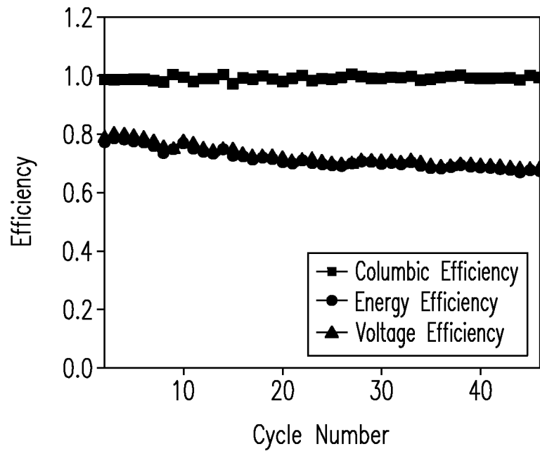
Fig. 10A
